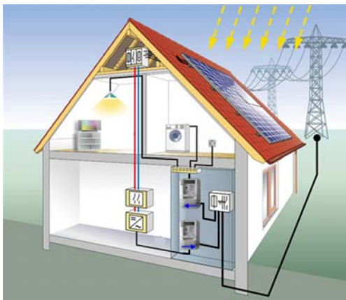
Einspeisung Komplettmenge
