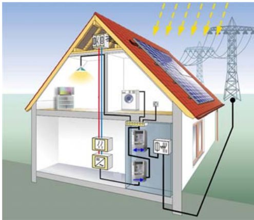
Einspeisung Überschussmenge
